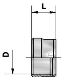
Изобр. 1 Врезное кольцо с 1 кромкой
