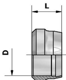
Изобр. 2 Врезное кольцо с 2 кромками
